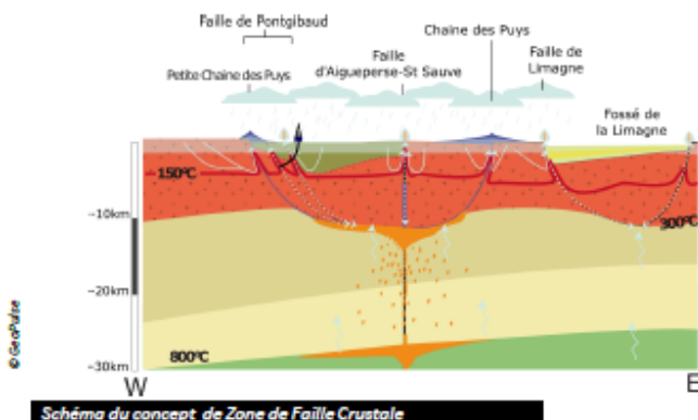
Schéma du concept de Zone de Faille Crustale
