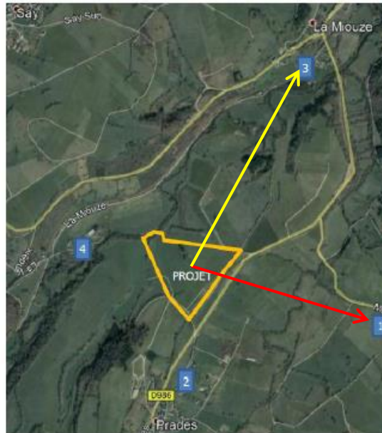
Figure 1 : Localisation des points de mesure acoustique (Étude AIROPTA)
